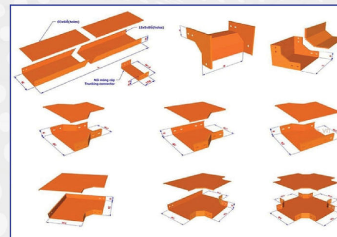
PHỤ KIỆN MÁNG CÁP TRUNKING ACCESSORIES
